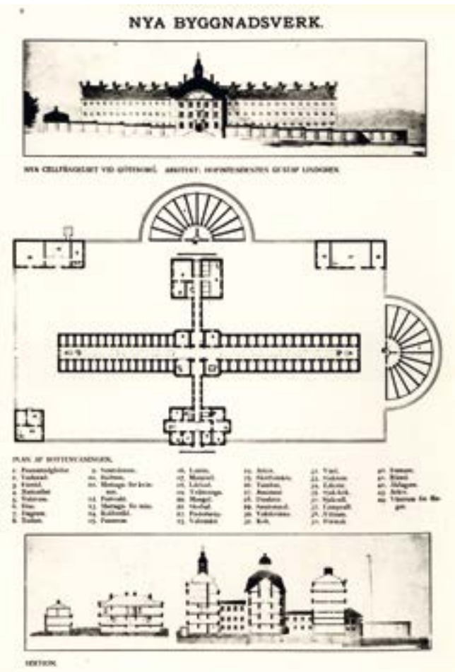
Ursprunglig Planritning för Härlanda fängelse Tillhör Göteborgs Stadsmuseum.
